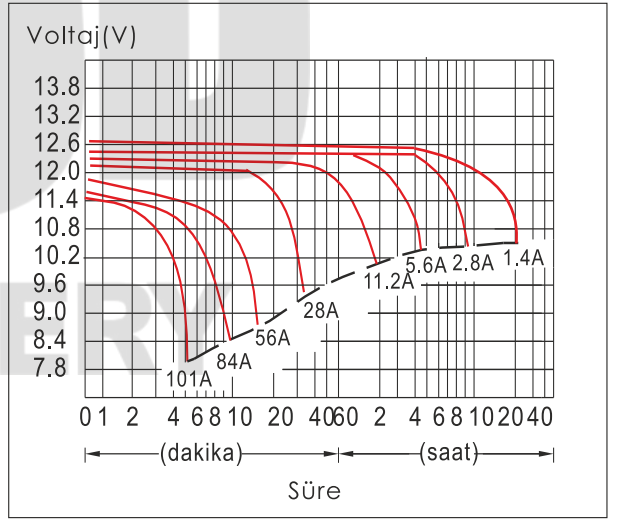
25°C(77°F) 'de Sabit Akım(Amper) ve Sabit Güç(Watt) Deşarj Tablosu
